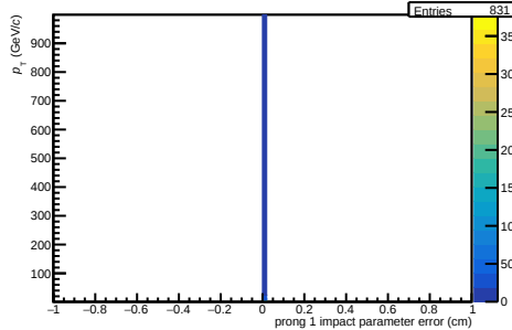
/hf-task-1c/Data/hImpParErrProng1VsPt NEW
