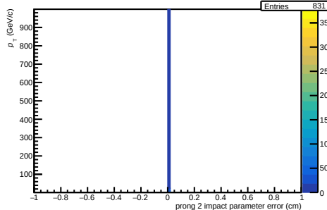
/hf-task-1c/Data/hImpParErrProng2VsPt NEW
