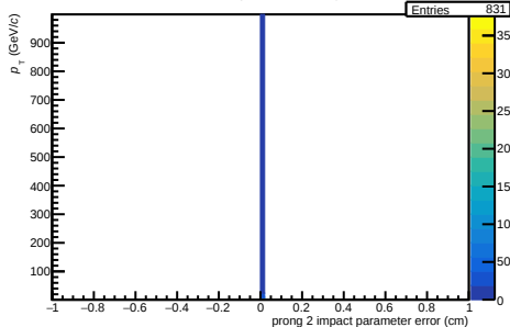
/hf-task-1c/Data/hImpParErrProng2VsPt OLD
