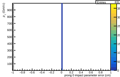
/hf-task-1c/Data/hImpParErrProng0VsPt NEW
