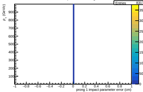
/hf-task-1c/Data/hImpParErrProng1VsPt OLD
