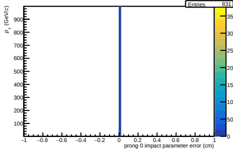
/hf-task-1c/Data/hImpParErrProng0VsPt OLD
