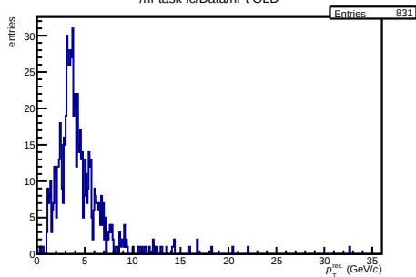
/hf-task-1c/Data/hPtProng0 OLD
