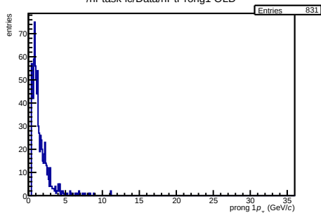
/hf-task-1c/Data/hPtProng1 OLD
